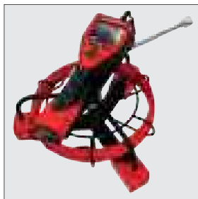
3 Модуль Pipe 25/16 Длина кабеля: 16 м Рабочий диапазон: до Ø 100 мм
